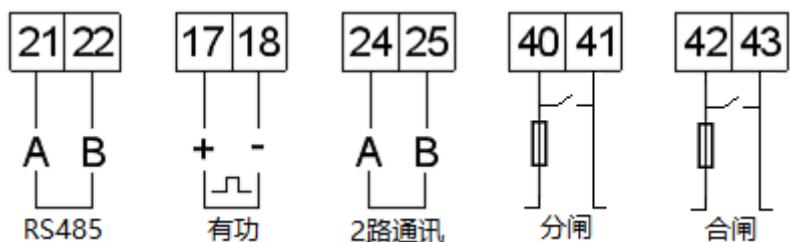
辅助功能 Auxiliary function
