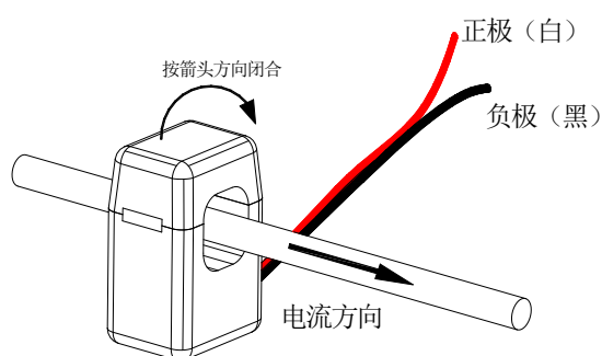
ACR10R-D10、D16 系列
