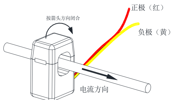
ACR10R-D24、36 系列
