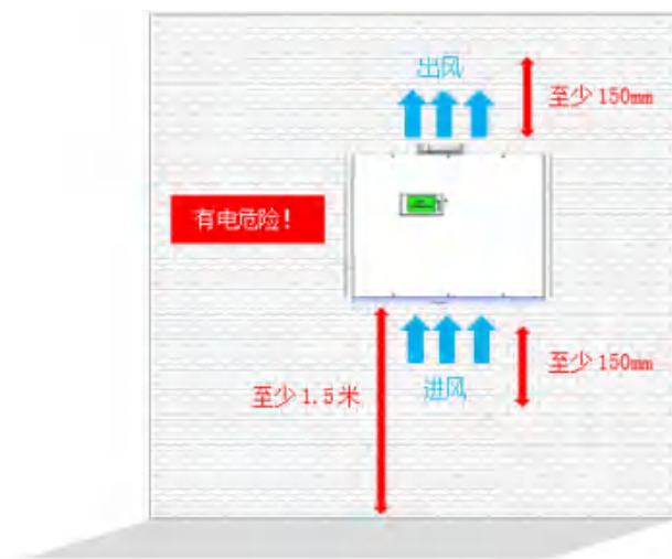
图6-3 立柜式安装空间要求示意图
