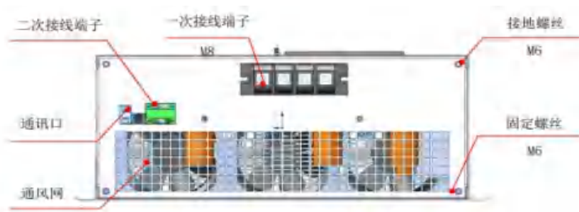
图4-15 50A/75A壁挂式模块顶部
