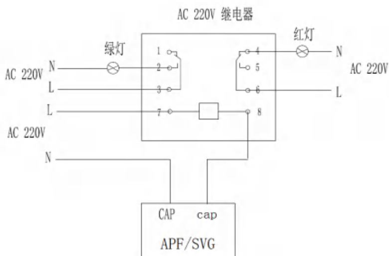
图 6-22 状态指示灯接口示意图
