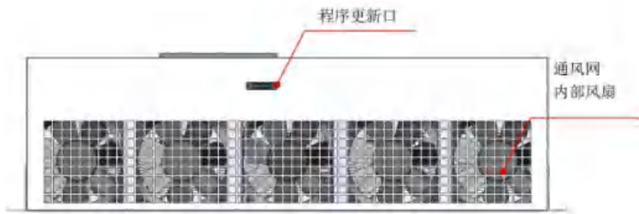
图4-11 150A/100A壁挂式模块底部
