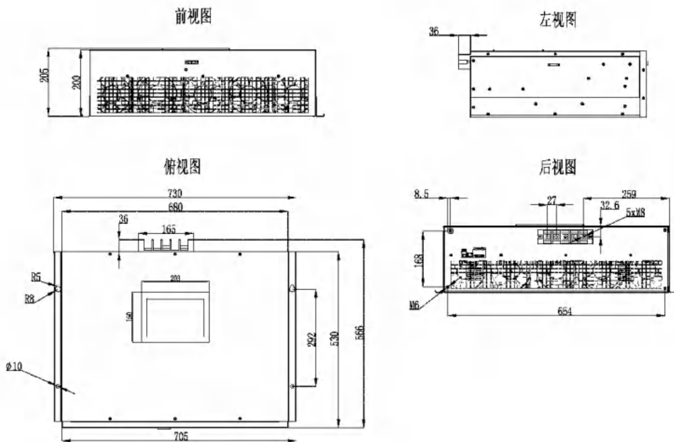
图4-12 150A/100A壁挂式模块尺寸图
