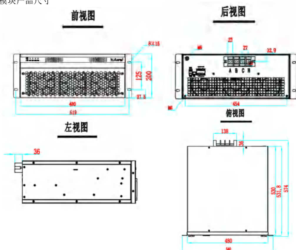
图4-5 75A抽屉式模块尺寸图
