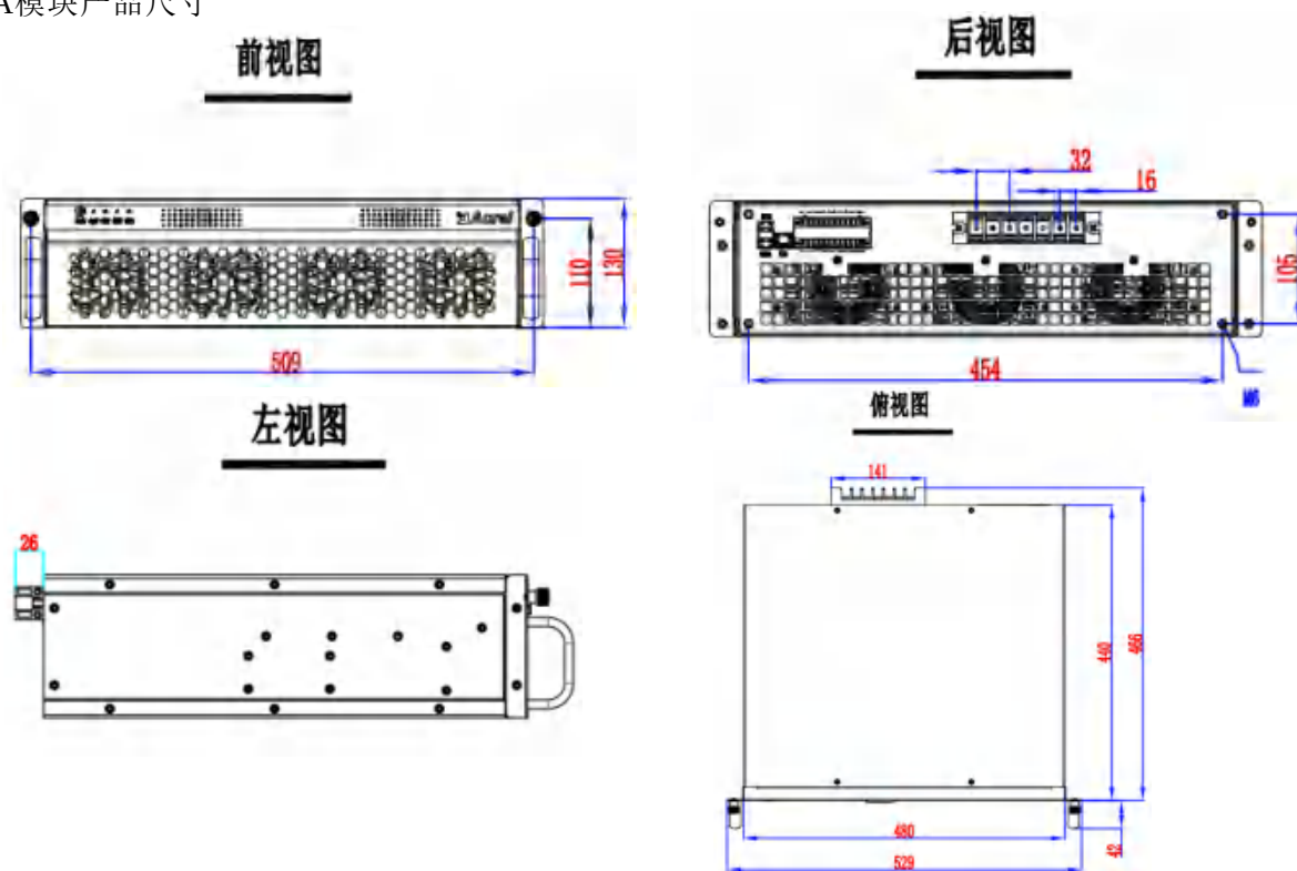
图4-7 30A抽屉式模块尺寸图
