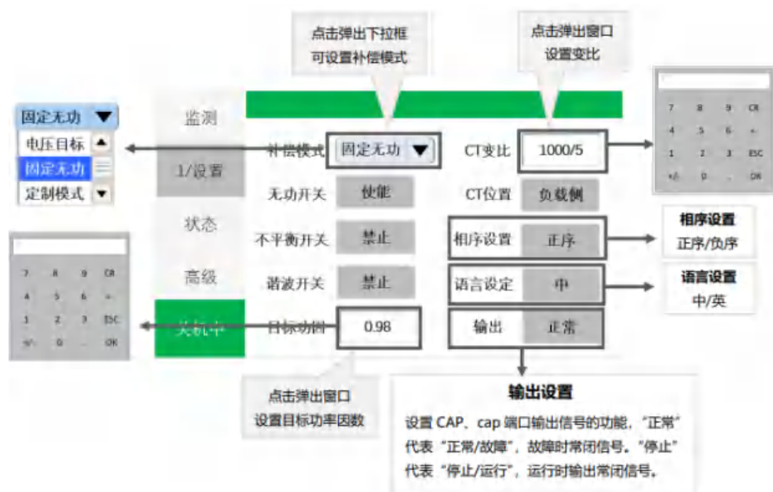
图 9-8 设置界面 1-基本设置
