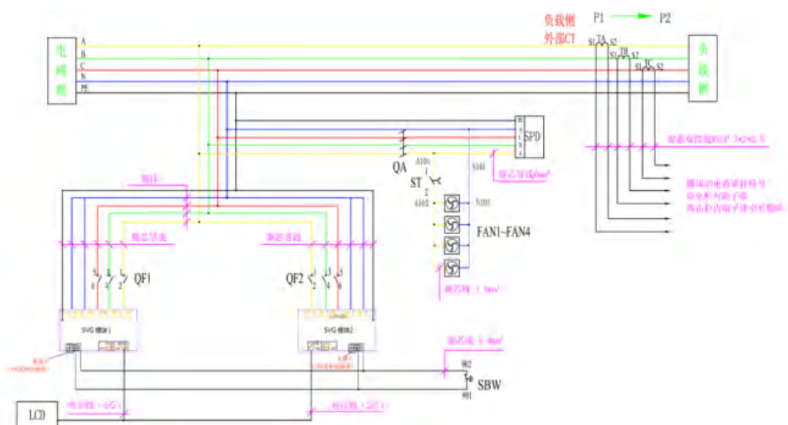
图 6-14 立柜式安装典型接线示意图
