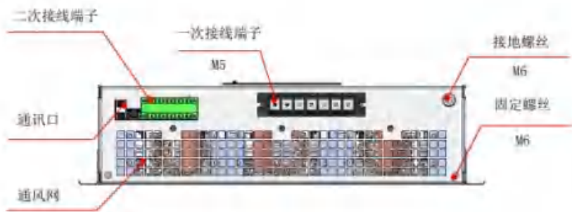
图4-20 30A壁挂式模块顶部
