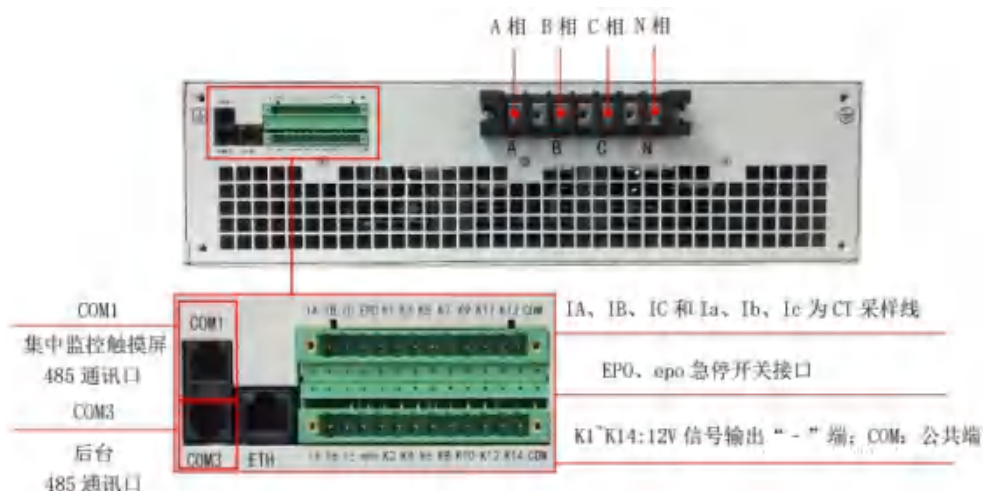
图4-25 30A模块端子示意图
