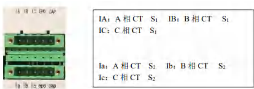
图 6-18 模块二次端子及 CT 线缆接入示意图
