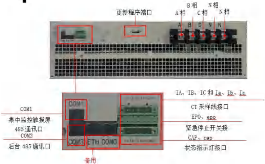
图4-22 200A模块端子示意图
