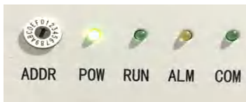
图4-26 拨码开关及状态指示灯示意图
