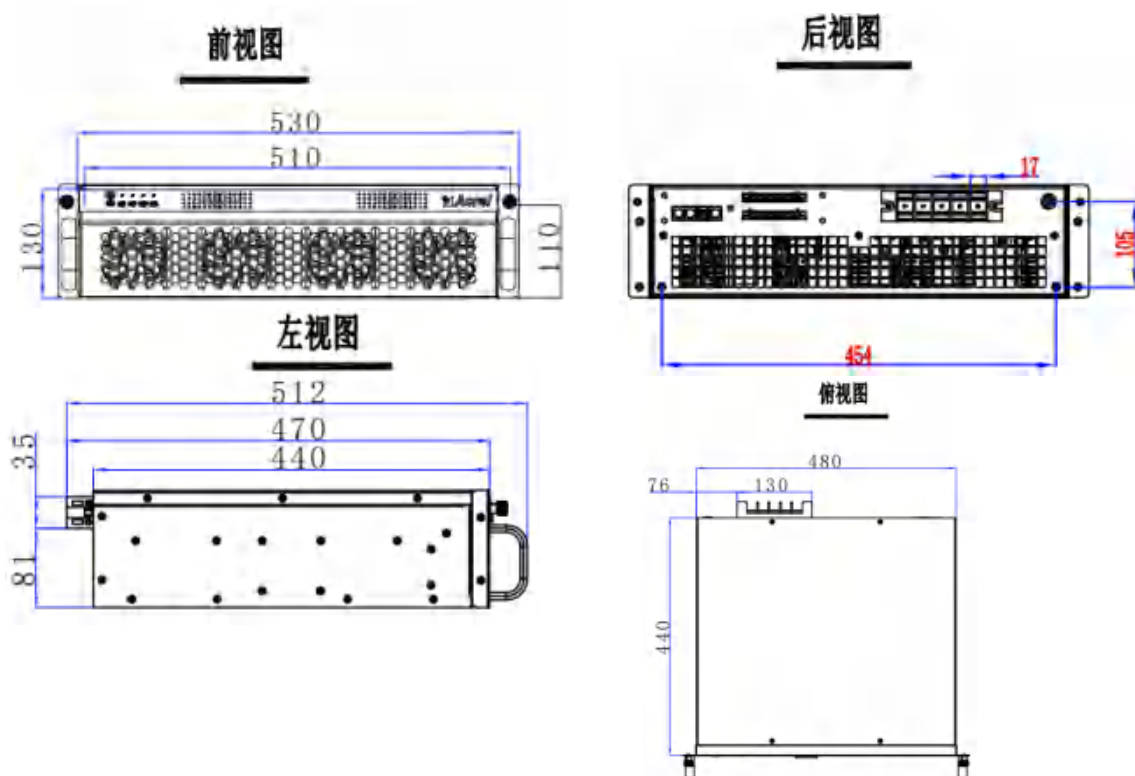
图4-6 50A抽屉式模块尺寸图
