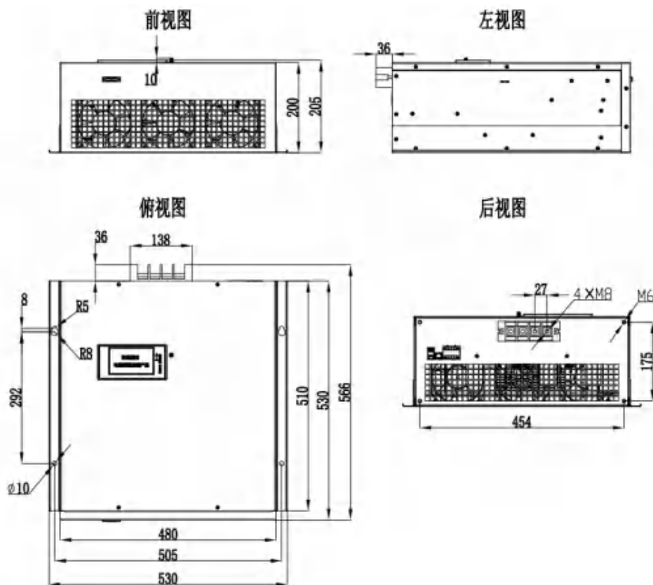
图4-17 50A/75A壁挂式模块尺寸图
