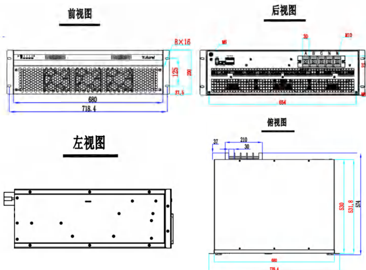
图4-4 200A/150A/100A抽屉式模块尺寸图
