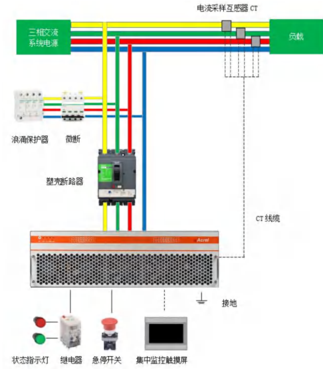
图5-1 ANAPF单模块系统连接图
