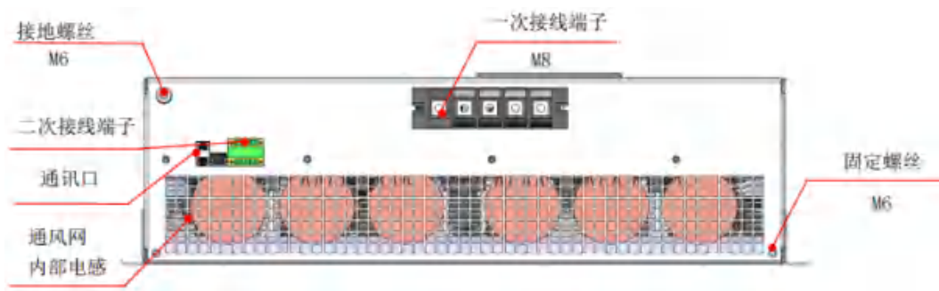
图4-10 150A/100A壁挂式模块顶部
