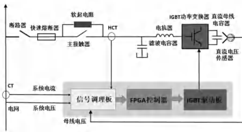
图3-2 ANAPF 内部控制原理图
