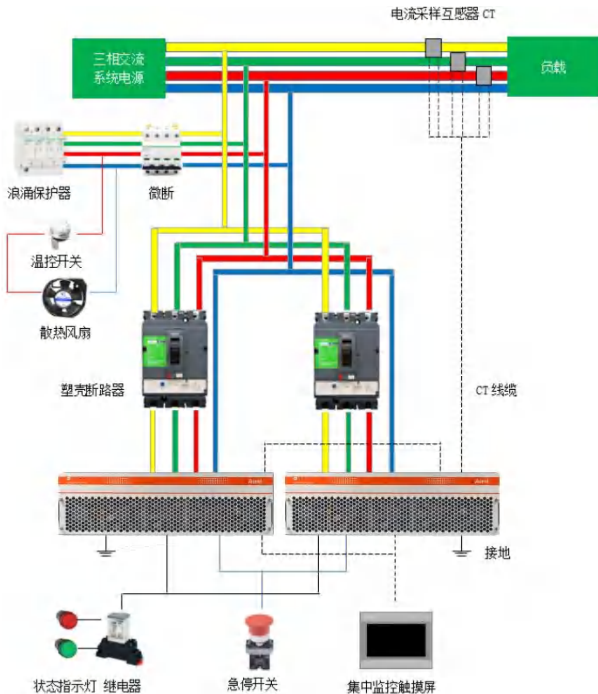
图5-2 ANAPF多模块系统并机连接图
