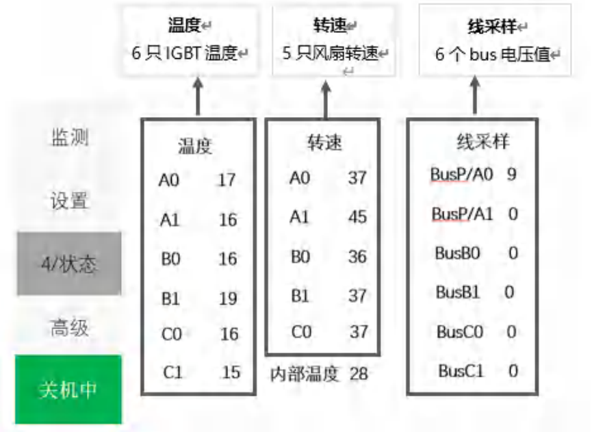
图 9-14 状态界面 4-温度转速采样状态
