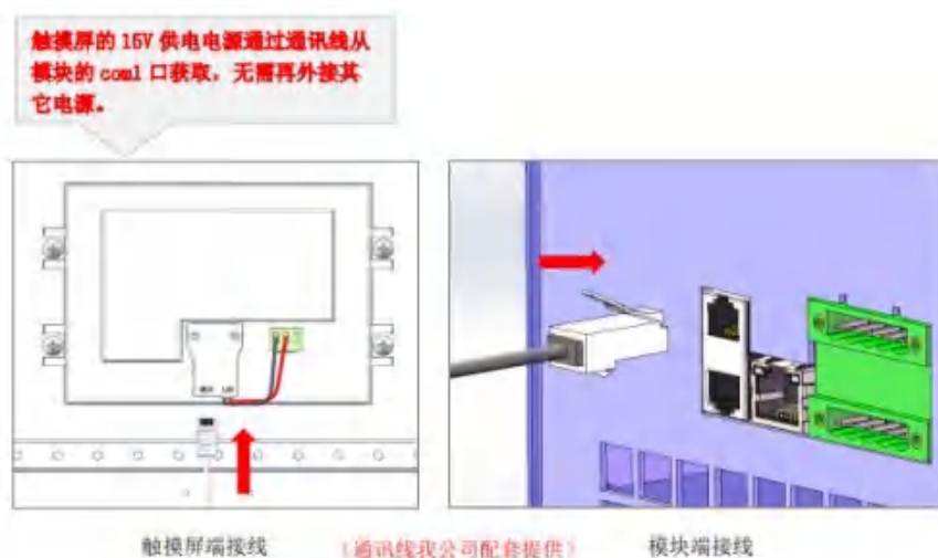
图 6-15 集中监控触摸屏通讯线接线示意图
