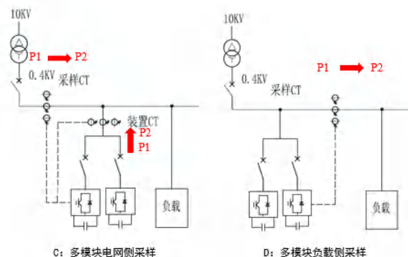
图 6-16 CT 采样方案示意图
