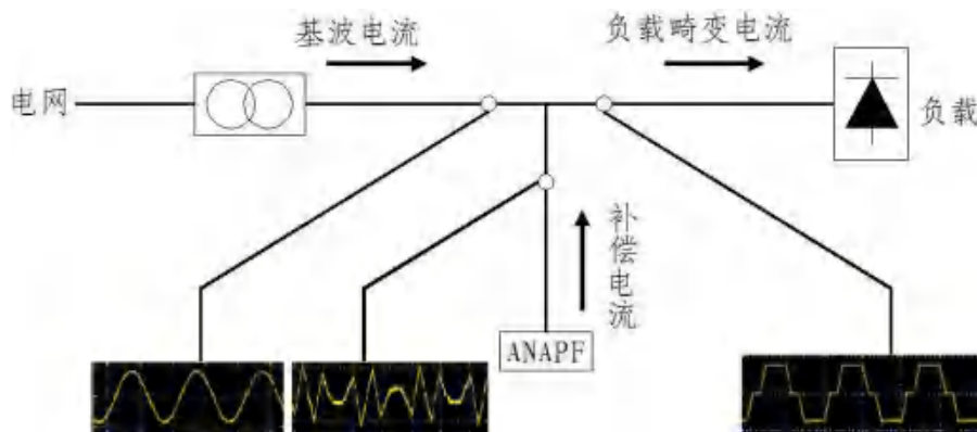
图3-1 ANAPF 工作原理图
