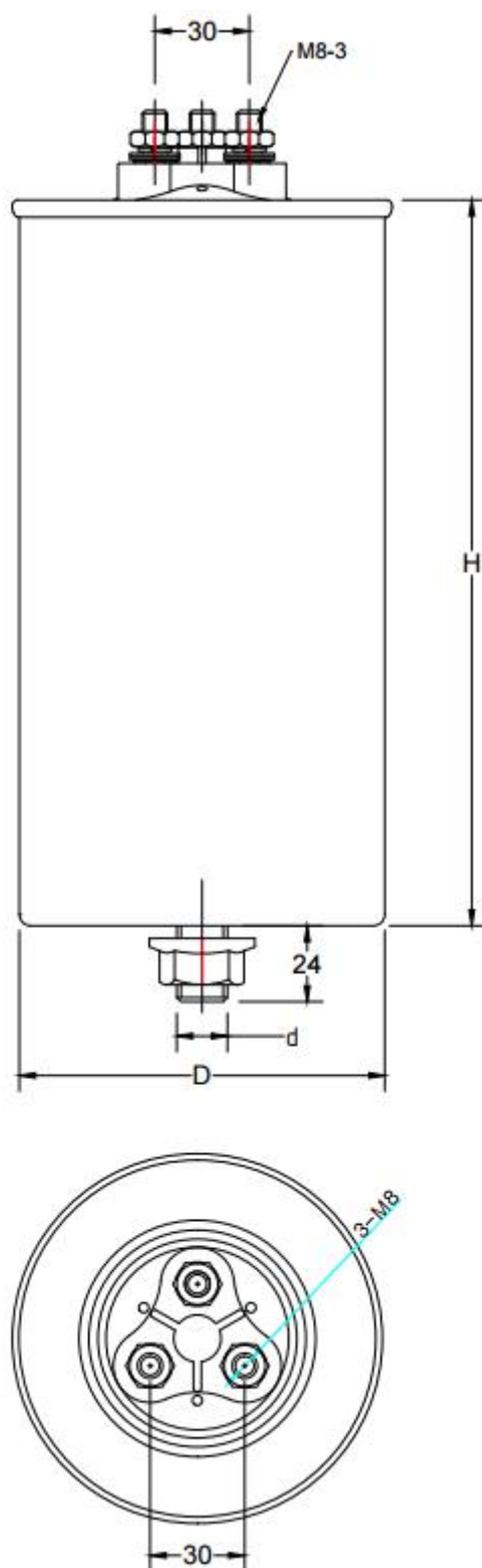
ANBSMJ 系列自愈式低压并联电容器（圆柱形、共补）外形尺寸图
