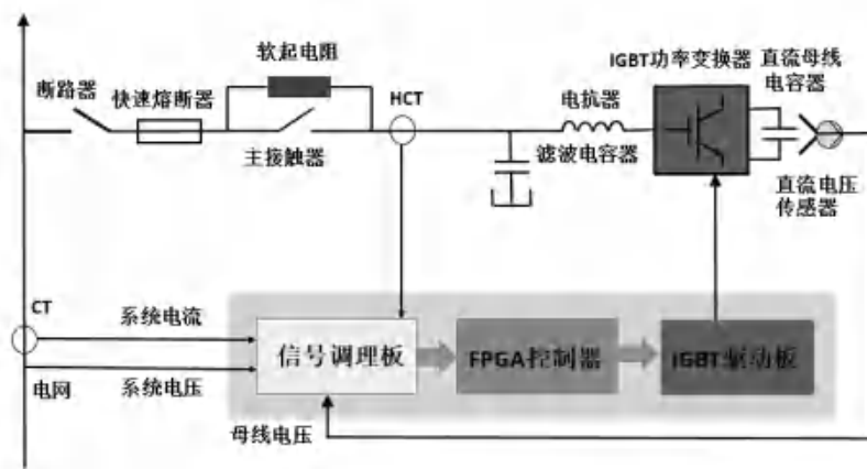
图3-2 ANSVG-G-A 内部控制原理图
