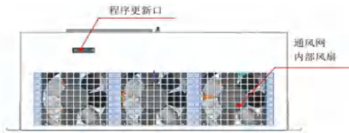
图4-16 50kvar-25A壁挂式模块底部
