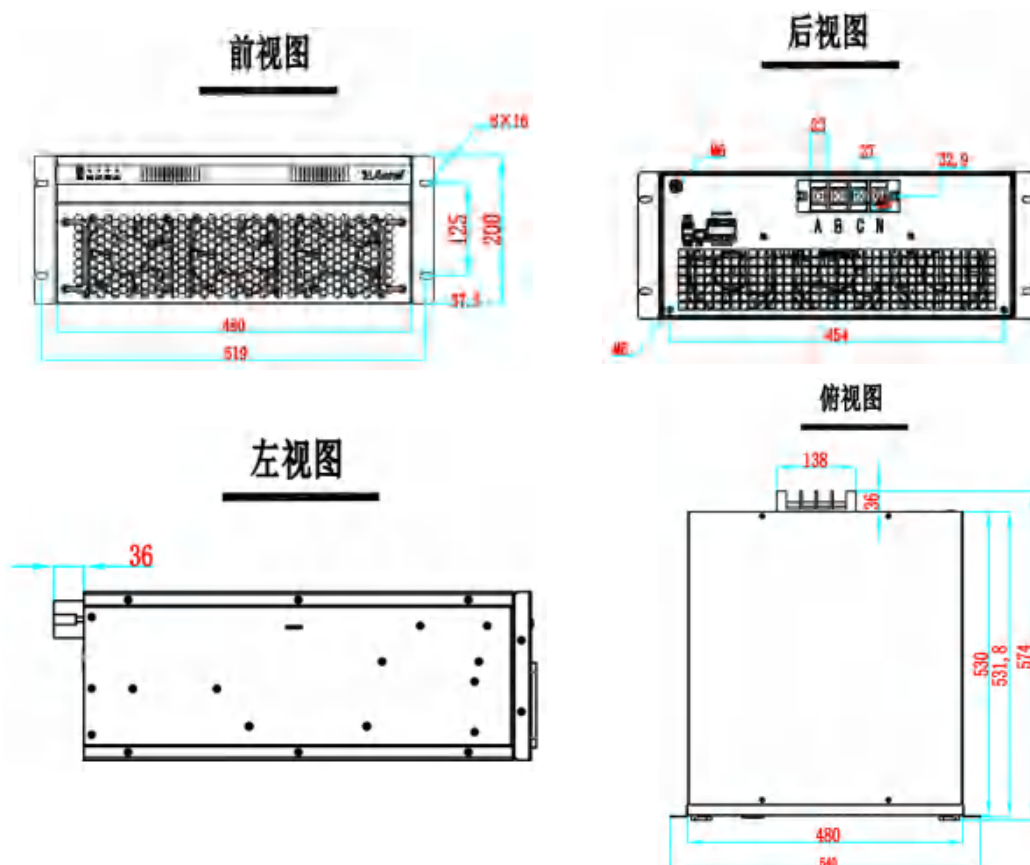
图4-6 50kvar-25A抽屉式模块尺寸图
