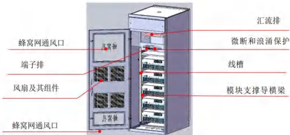
图6-7 整柜示意图（背面）
