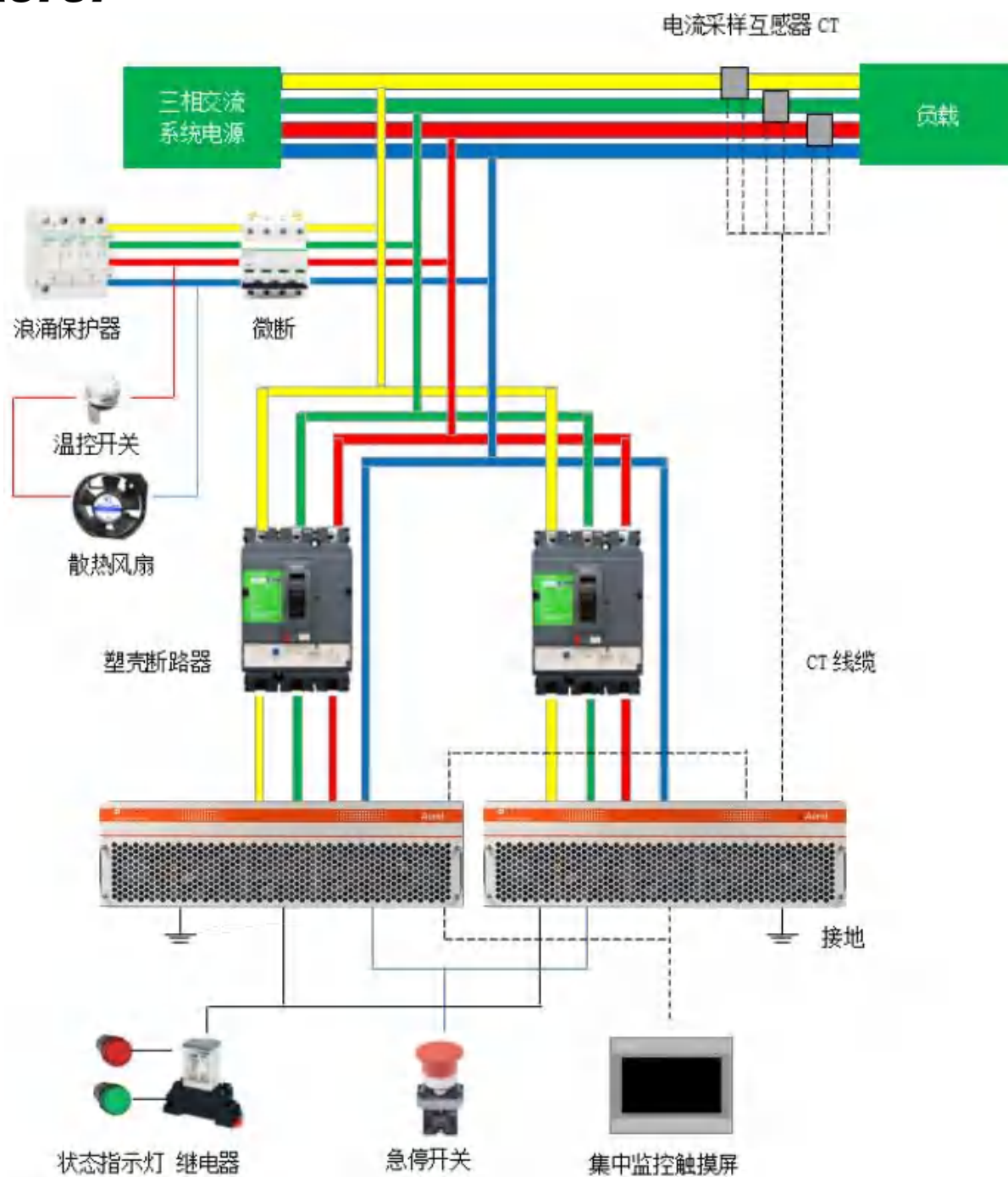
图5-2 ANSVG-G-A多模块系统并机连接图
