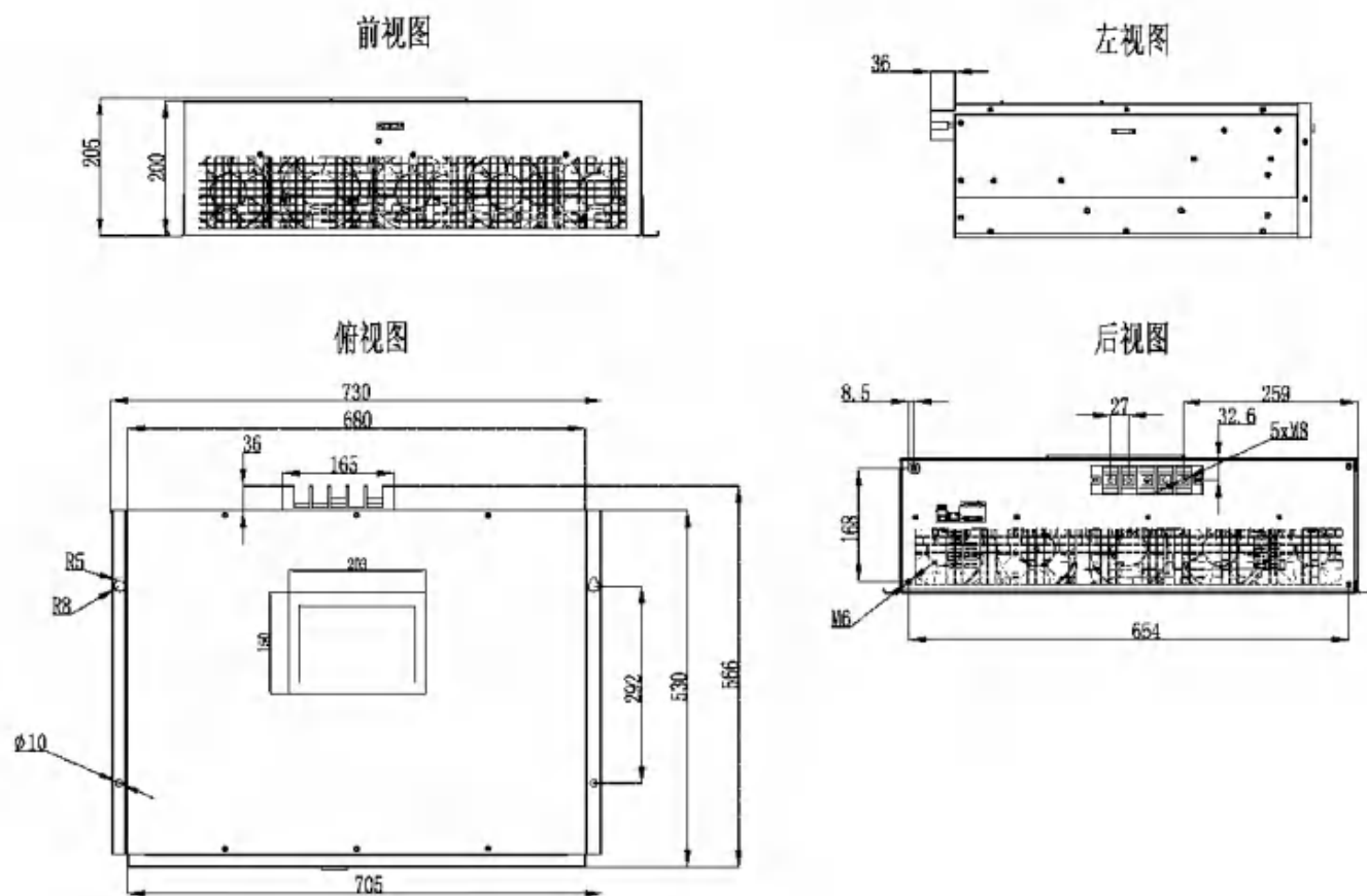
图4-12 75kvar-37.5A/100kvar-50A壁挂式模块尺寸图
