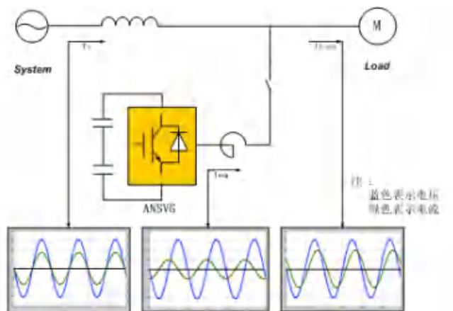
图3-1 ANSVG-G-A 工作原理图
