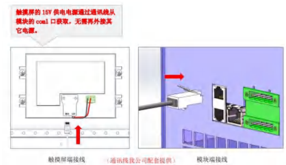
图 6-15 集中监控触摸屏通讯线接线示意图
