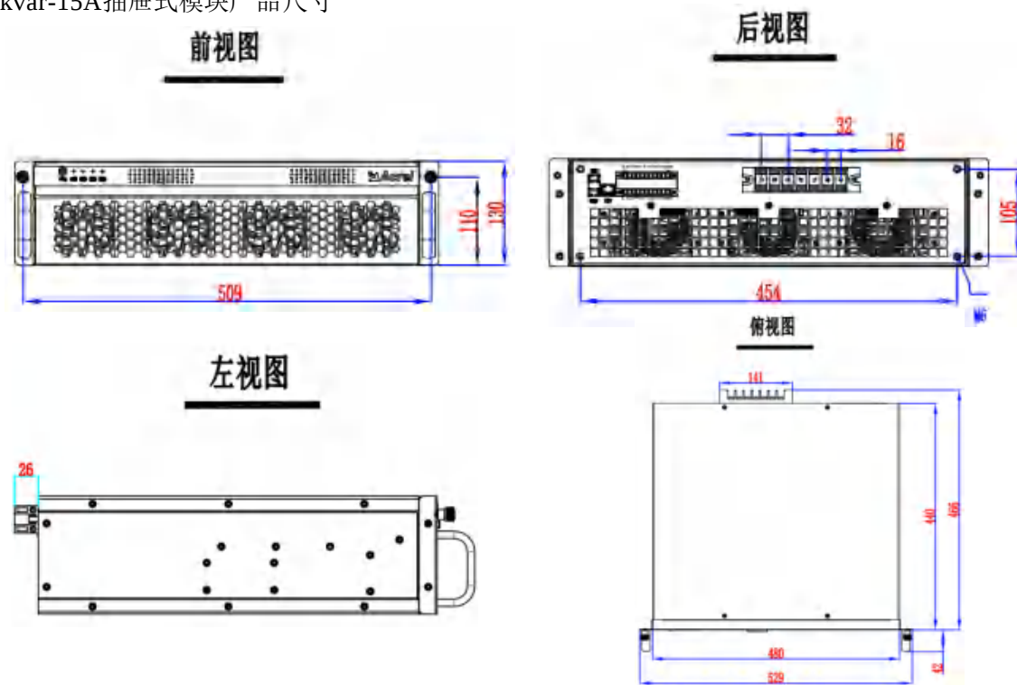
图4-7 30kvar-15A抽屉式模块尺寸图
