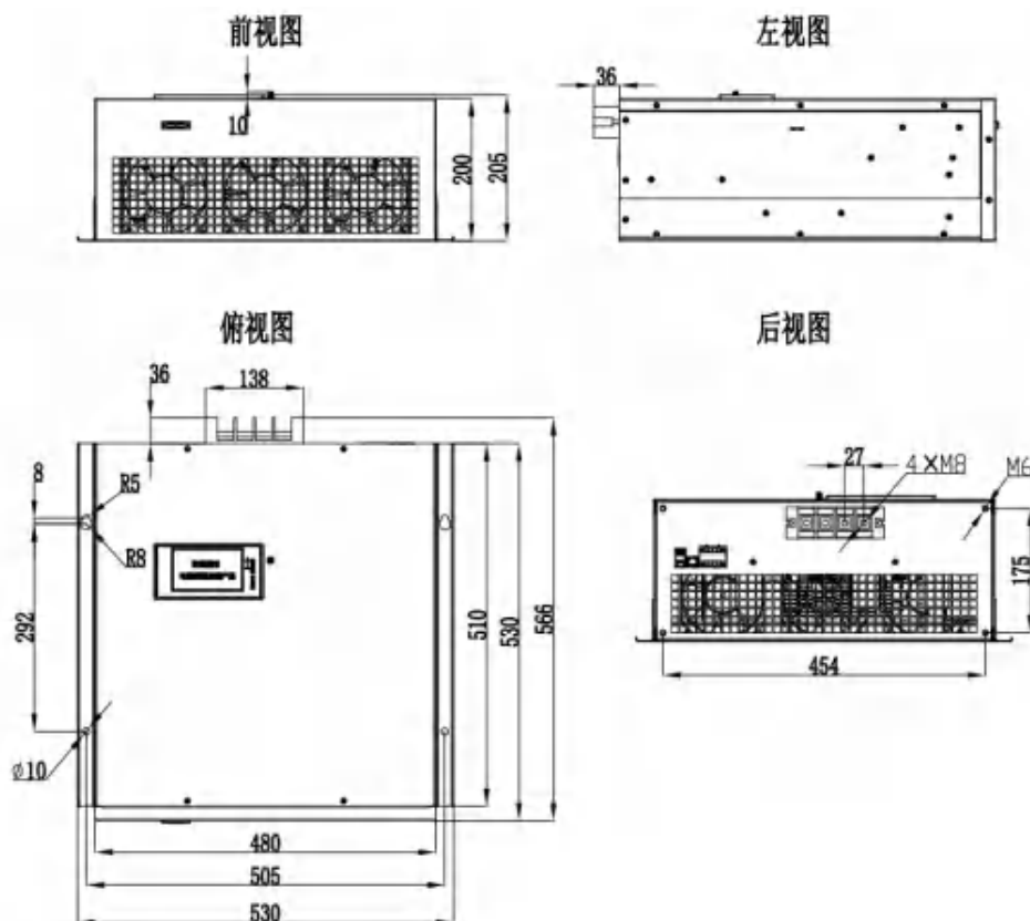
图4-17 50kvar-25A壁挂式模块尺寸图
