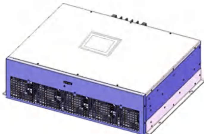
图4-8 75kvar-37.5A/100kvar-50A壁挂式模块外观
