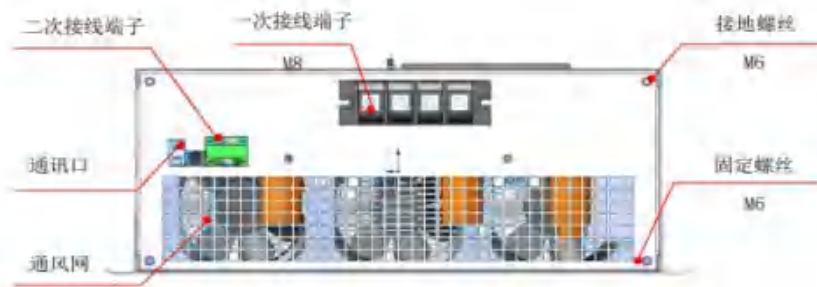
图4-15 50kvar-25A壁挂式模块顶部
