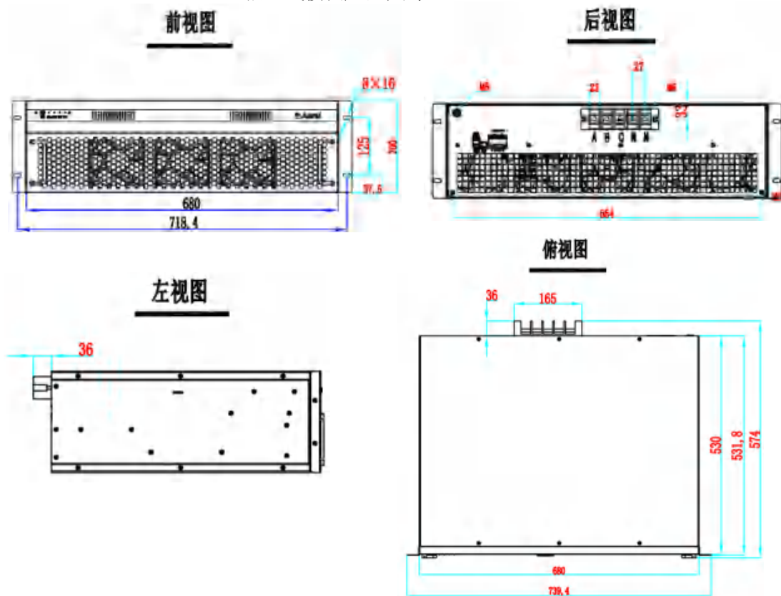
图4-5 75kvar-37.5A/100kvar-50A抽屉式模块尺寸图
