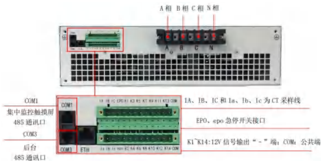
图4-25 30kvar-15A模块端子示意图
