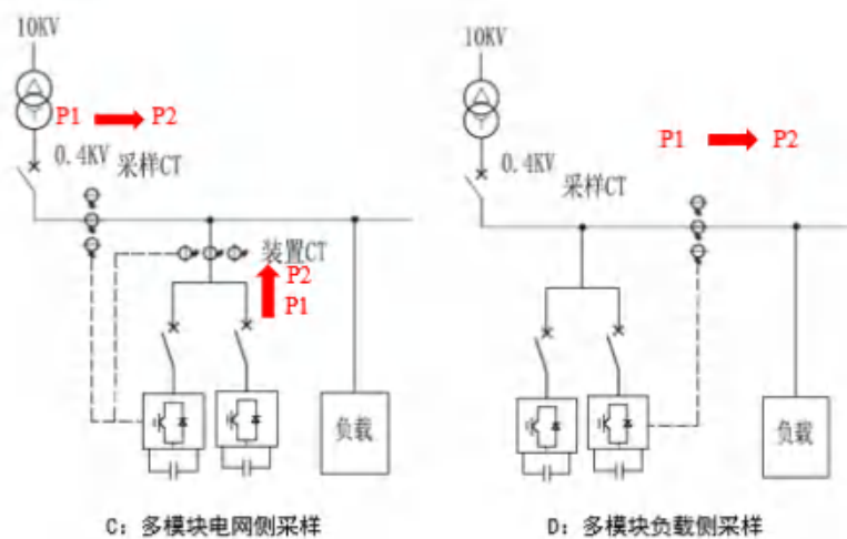
图 6-16 CT 采样方案示意图
