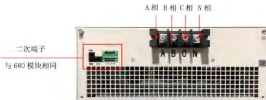
图4-24 50kvar-25A模块端子示意图
