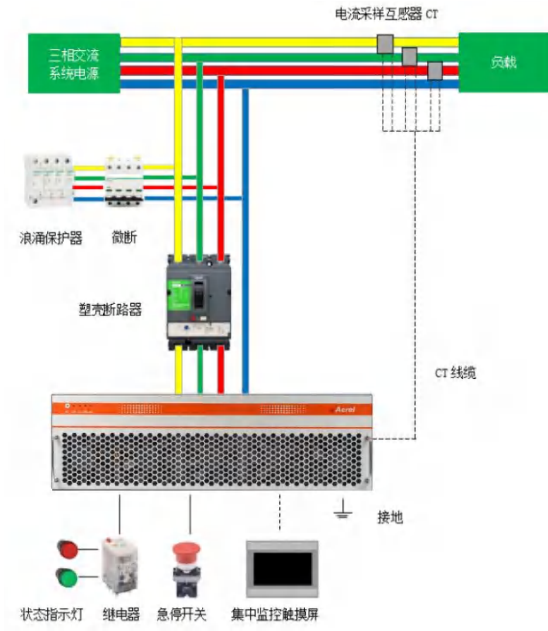
图5-1 ANSVG-G-A单模块系统连接图
