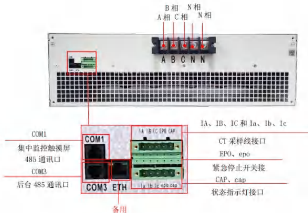
图4-23 75kvar-37.5A/100kvar-50A模块端子示意图
