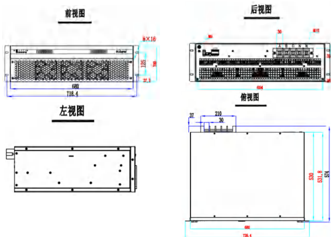
图4-4 150kvar-75A抽屉式模块尺寸图
