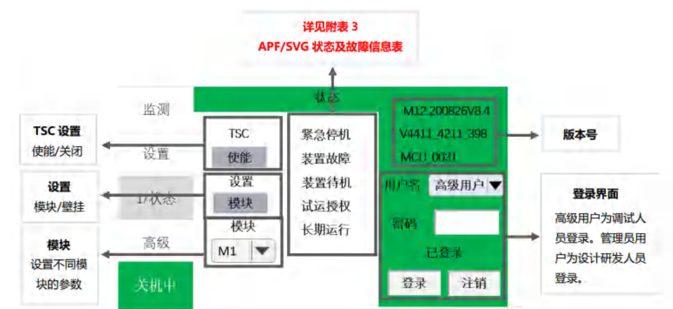
图 9-11 状态界面 1-登录及模块状态
