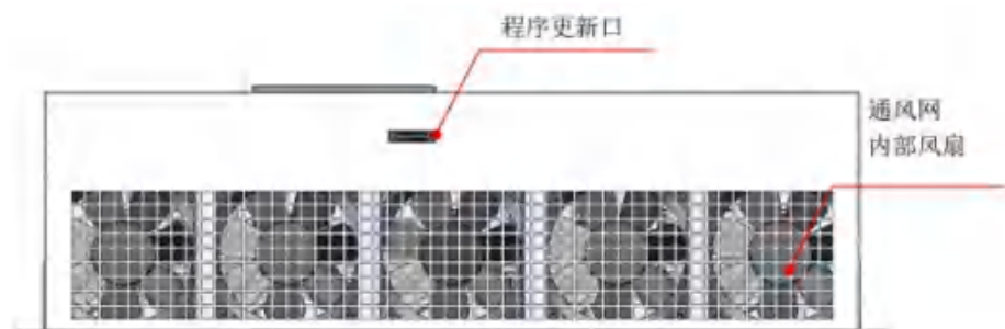
图4-11 75kvar-37.5A/100kvar-50A壁挂式模块底部
