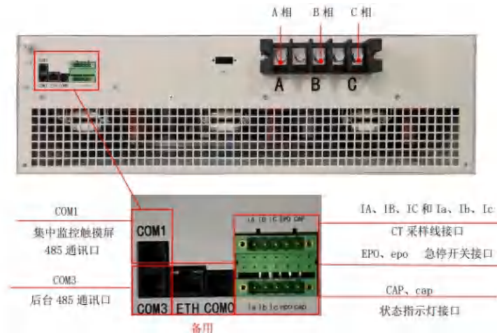
图4-26 100kvar-50A/50kvar-25A模块端子示意图
