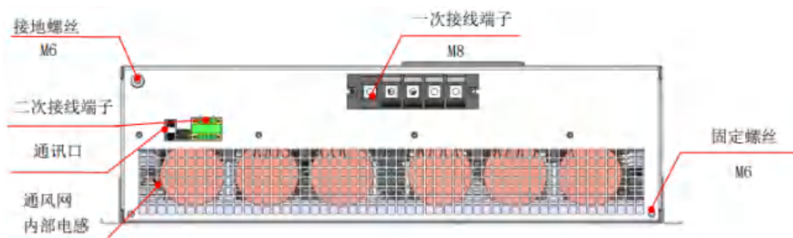
图4-9 75kvar-37.5A/100kvar-50A A壁挂式模块正面
