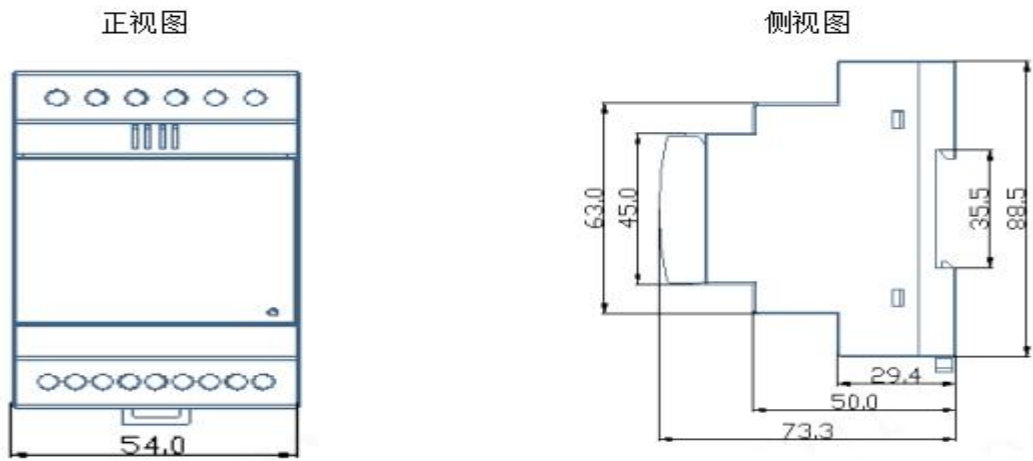
图 1.1 ARTM-D1 尺寸图
