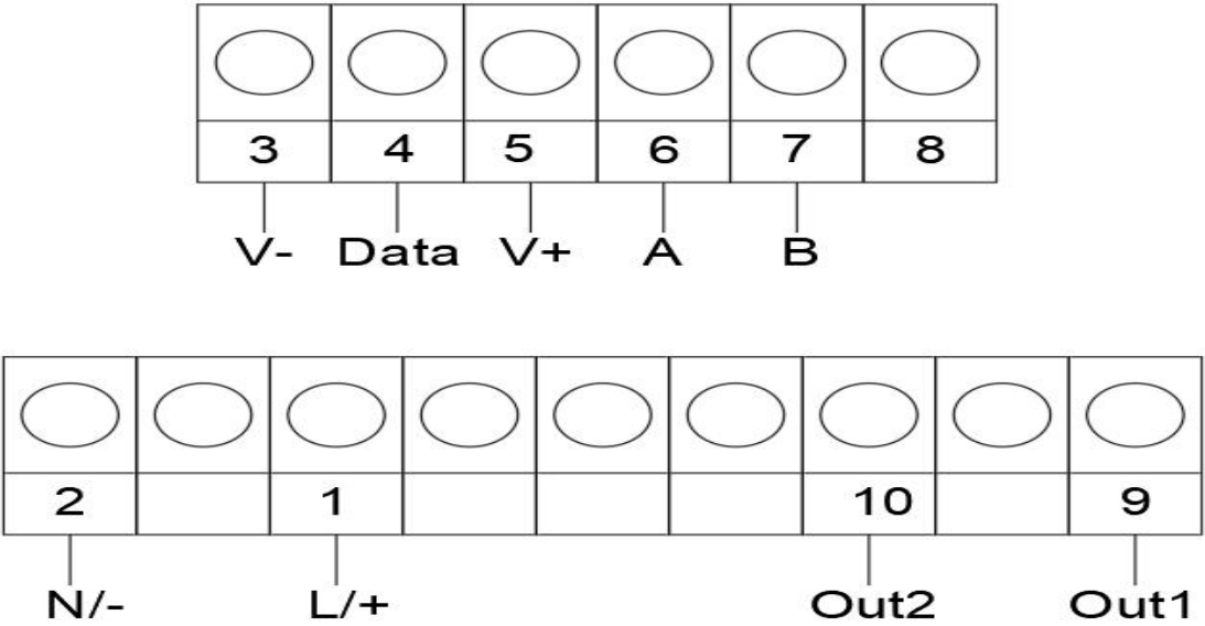
1.2 ARTM-D1 端子图
